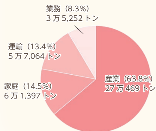
CO 2 部門別排出量 (2018 年)
