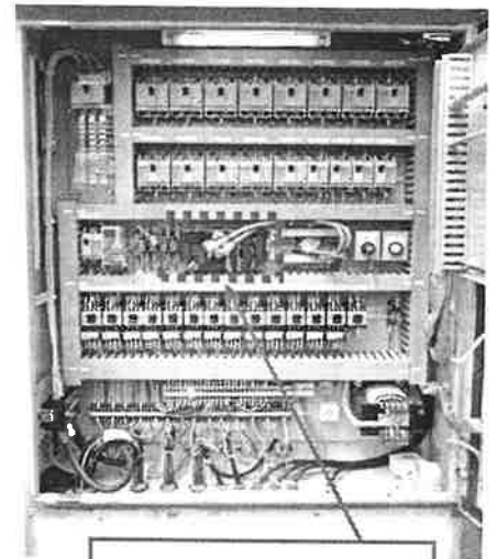
シーケンサー取替
