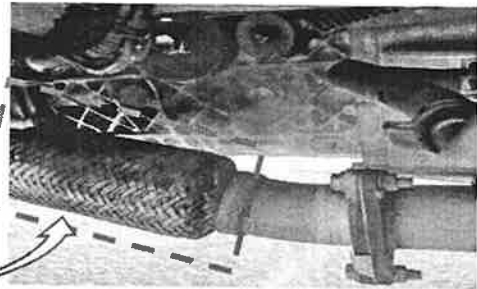
【メッシュ部分から白煙発生】
